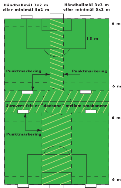
Fig. 2. Forslag til oppmerking av 4 baner på vanlige store baner (2. alt.)
